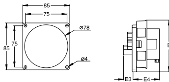
Ölçüler (mm)
