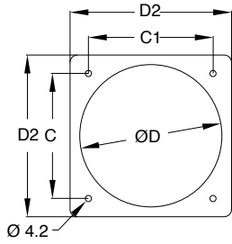
Ölçüler (mm)
