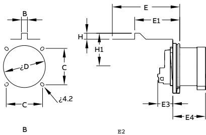
Ölçüler (mm)
