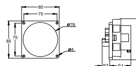
Ölçüler (mm)
