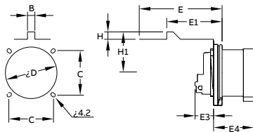
Ölçüler (mm)
